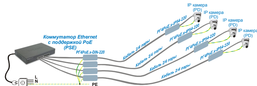
Пример использования PG4PoE.x-DIN-220 в паре с PG4PoE.x-IP54-220 на сети с применением технологии PoE (IEEE802.3af/at).
