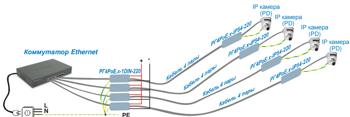
Пример использования PG4PoE.x-1DIN-220 в паре с PG4PoE.x-IP54-220 на сети с применением технологии PassivePoE.
