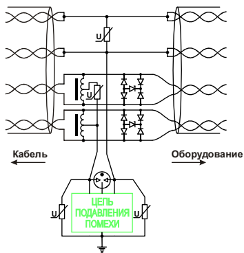
Модель Fast Ethernet (100 Мбит/С)
