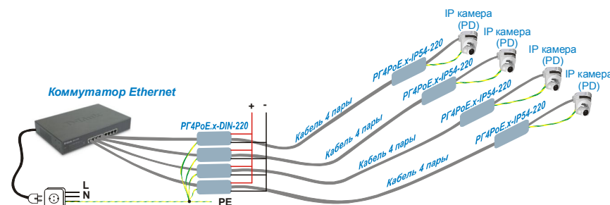
Пример использования PG4PoE.x-DIN-220 в паре с PG4PoE.x-IP54-220 на сети с применением технологии PassivePoE.
