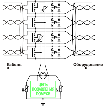
Модель Gigabit Ethernet (1000 Мбит/С)
