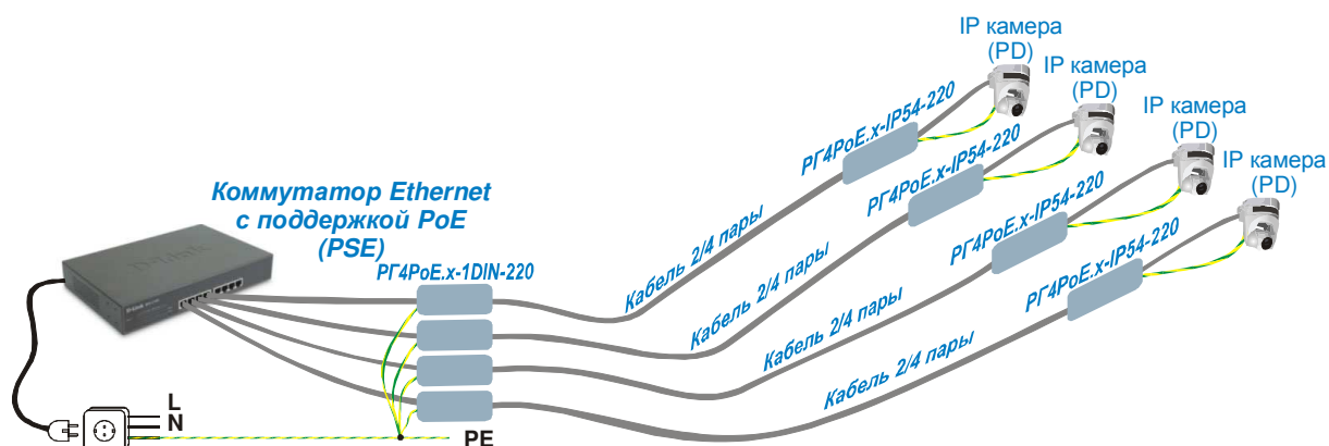
Пример использования PG4PoE.x-1DIN-220 в паре с PG4PoE.x-IP54-220 на сети с применением технологии PoE (IEEE802.3af/at).
